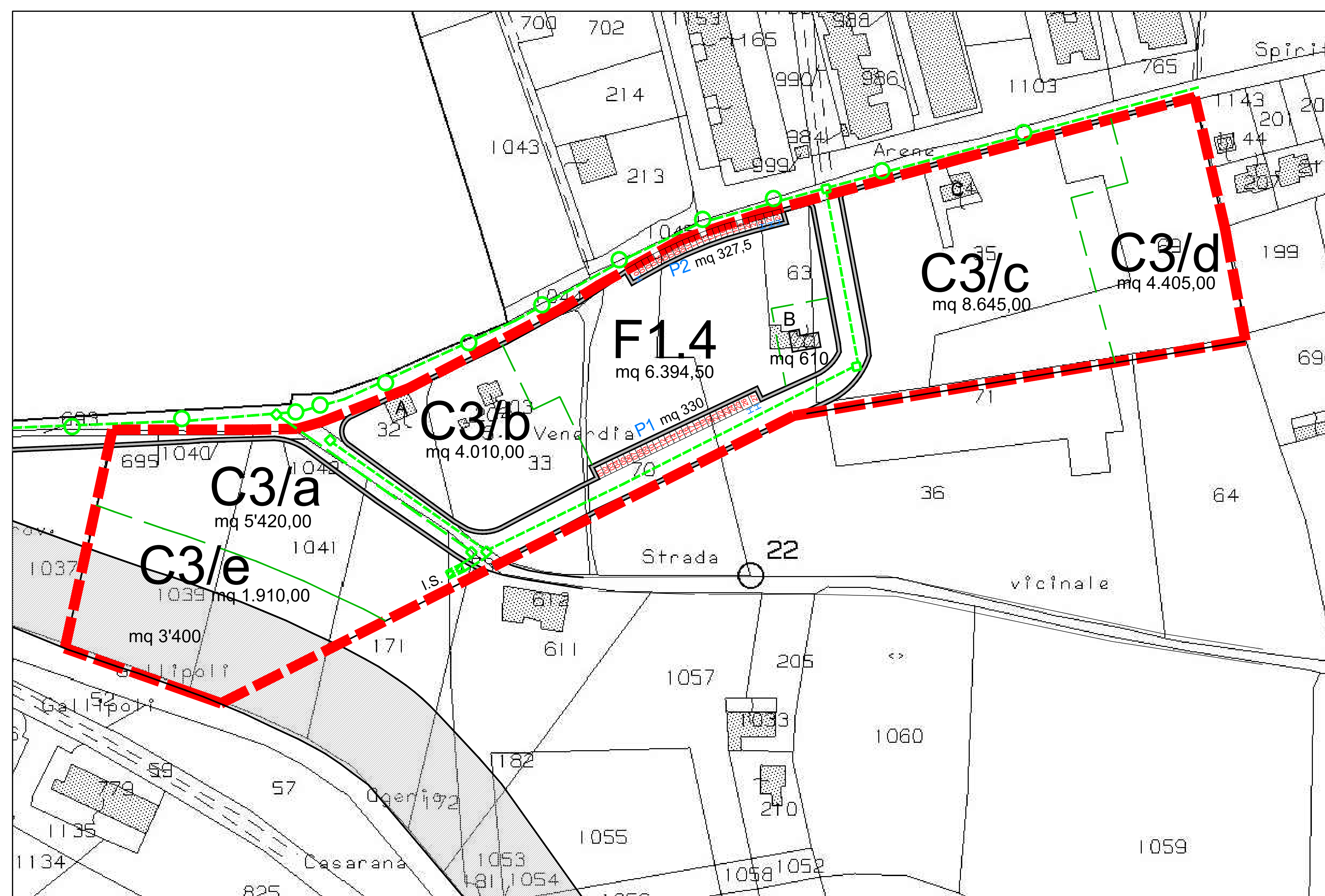
RETE FOGNANTE ACQUE NERE - rapp. 1 : 1000
