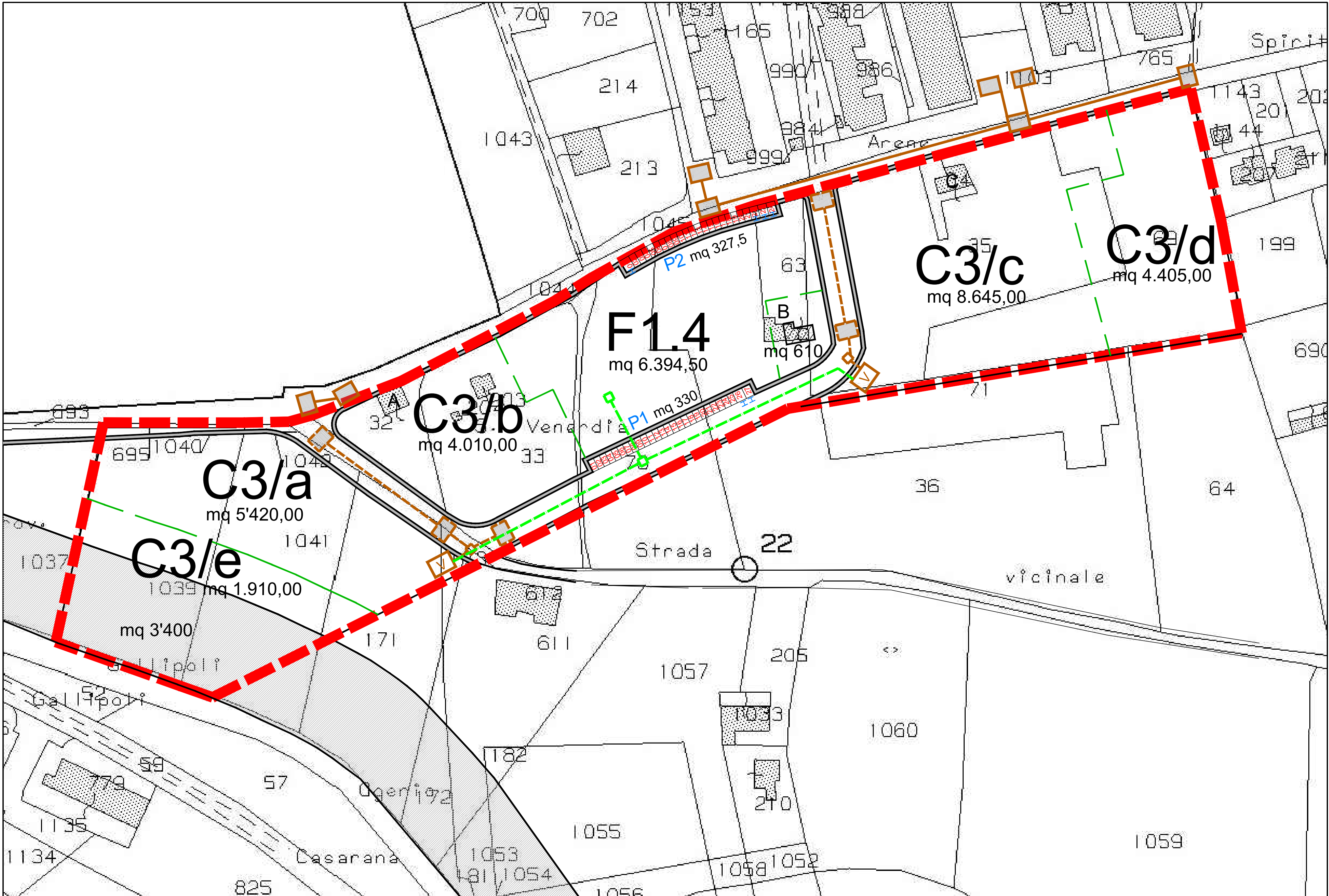
RETE FOGNANTE ACQUE PLUVIALI - rapp. 1 : 1000
