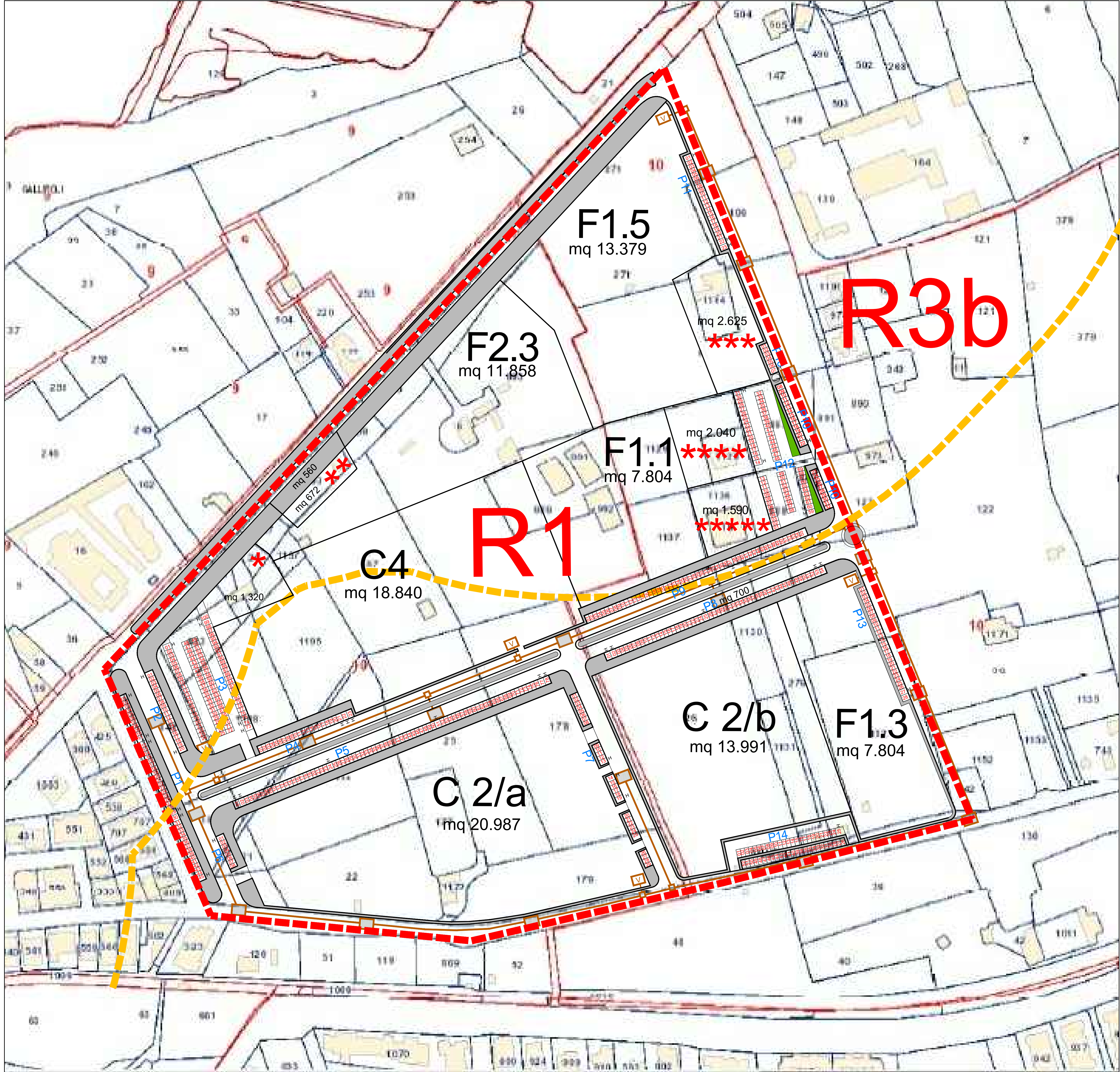
RETE FOGNANTE ACQUE PLUVIALI - rapp. 1 : 1000
