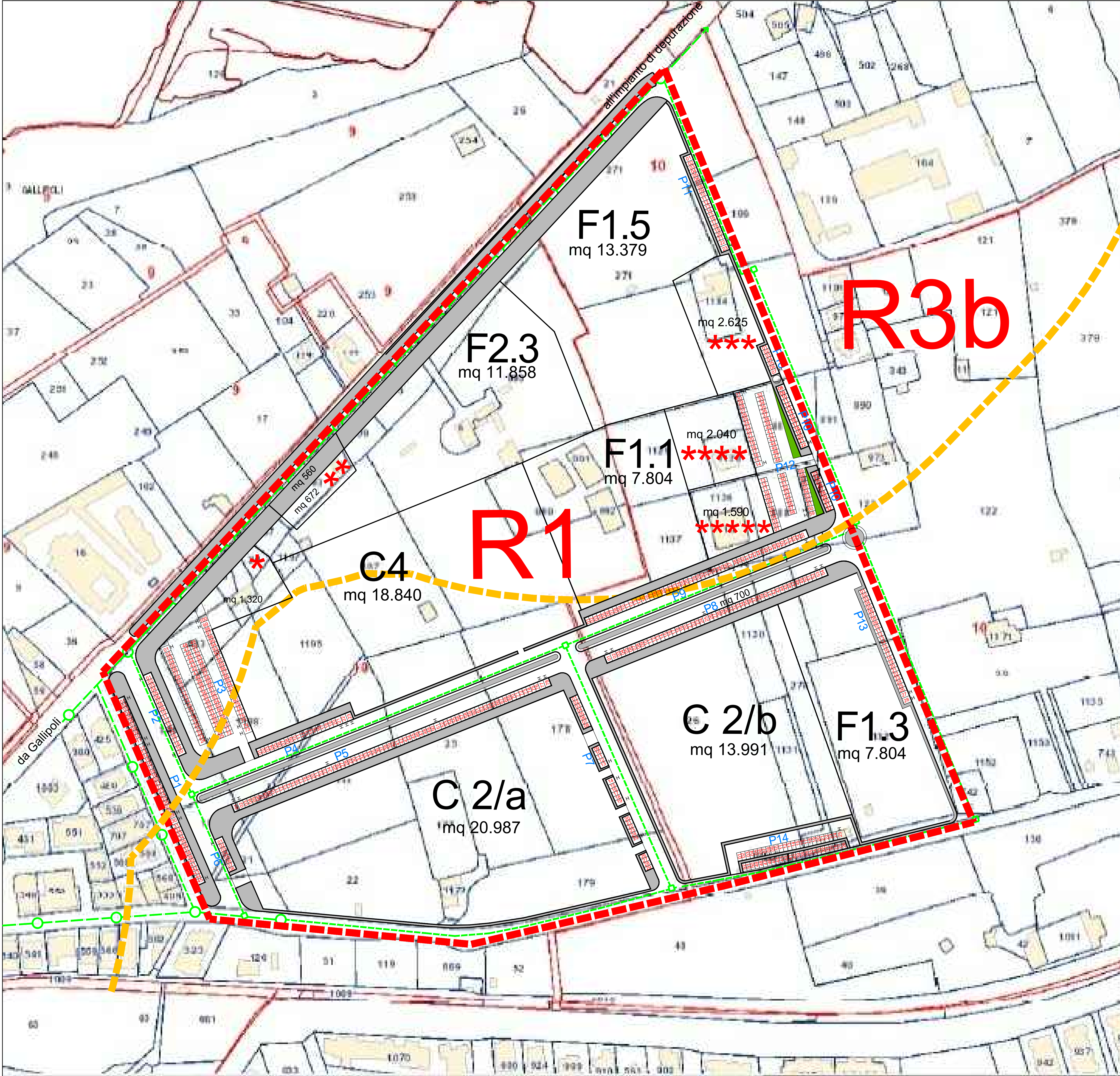
RETE FOGNANTE ACQUE NERE - rapp. 1 : 1000
