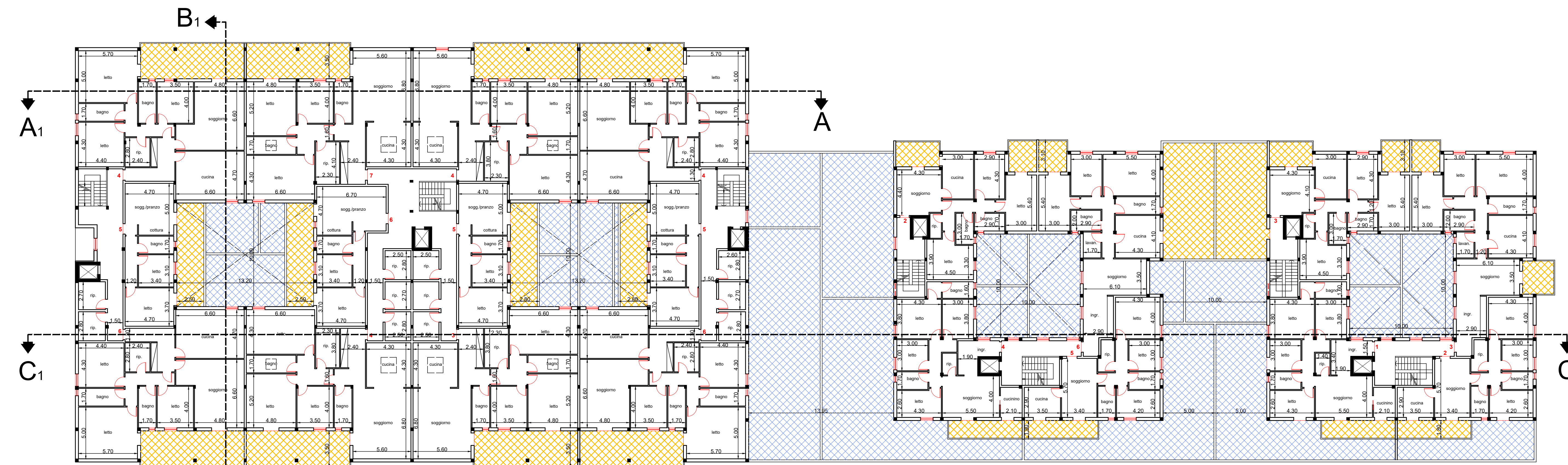
PIANO SECONDO - scala 1:200
