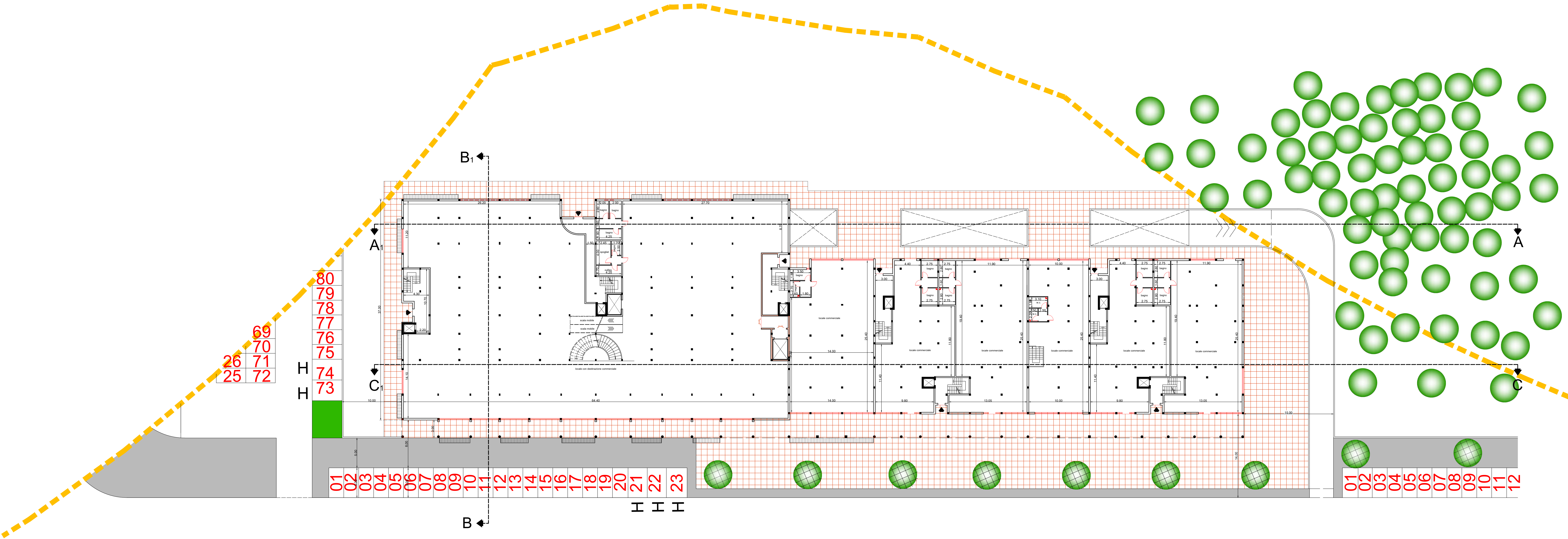
PIANO TERRA - scala 1:200
