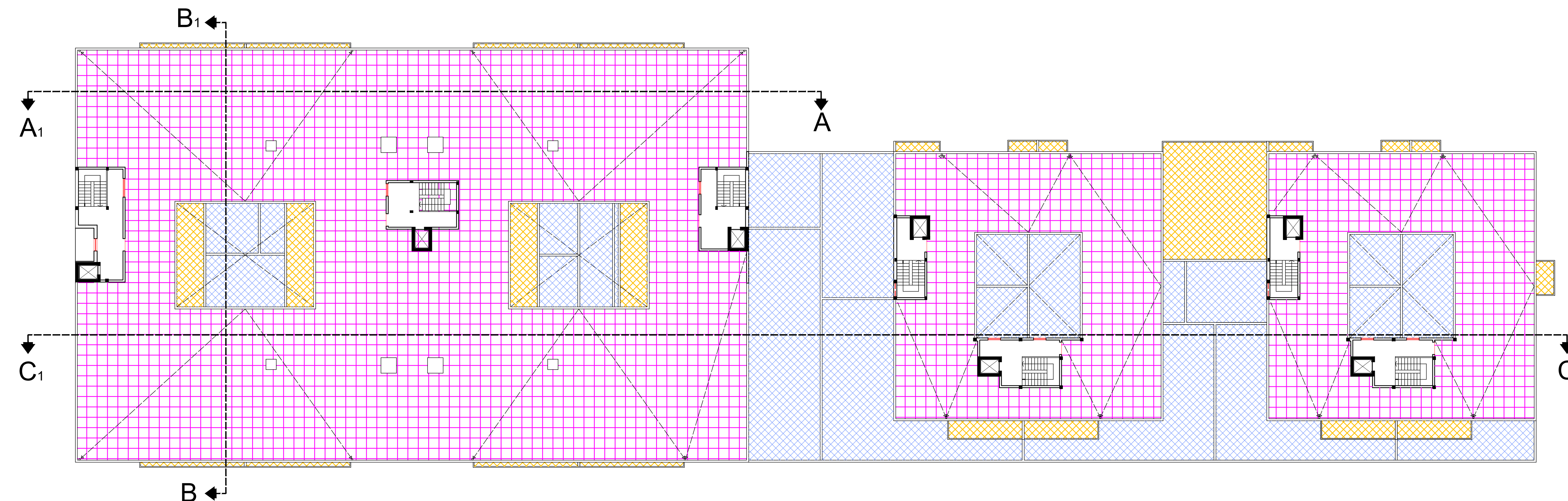
PIANO COPERTURA - scala 1:200
