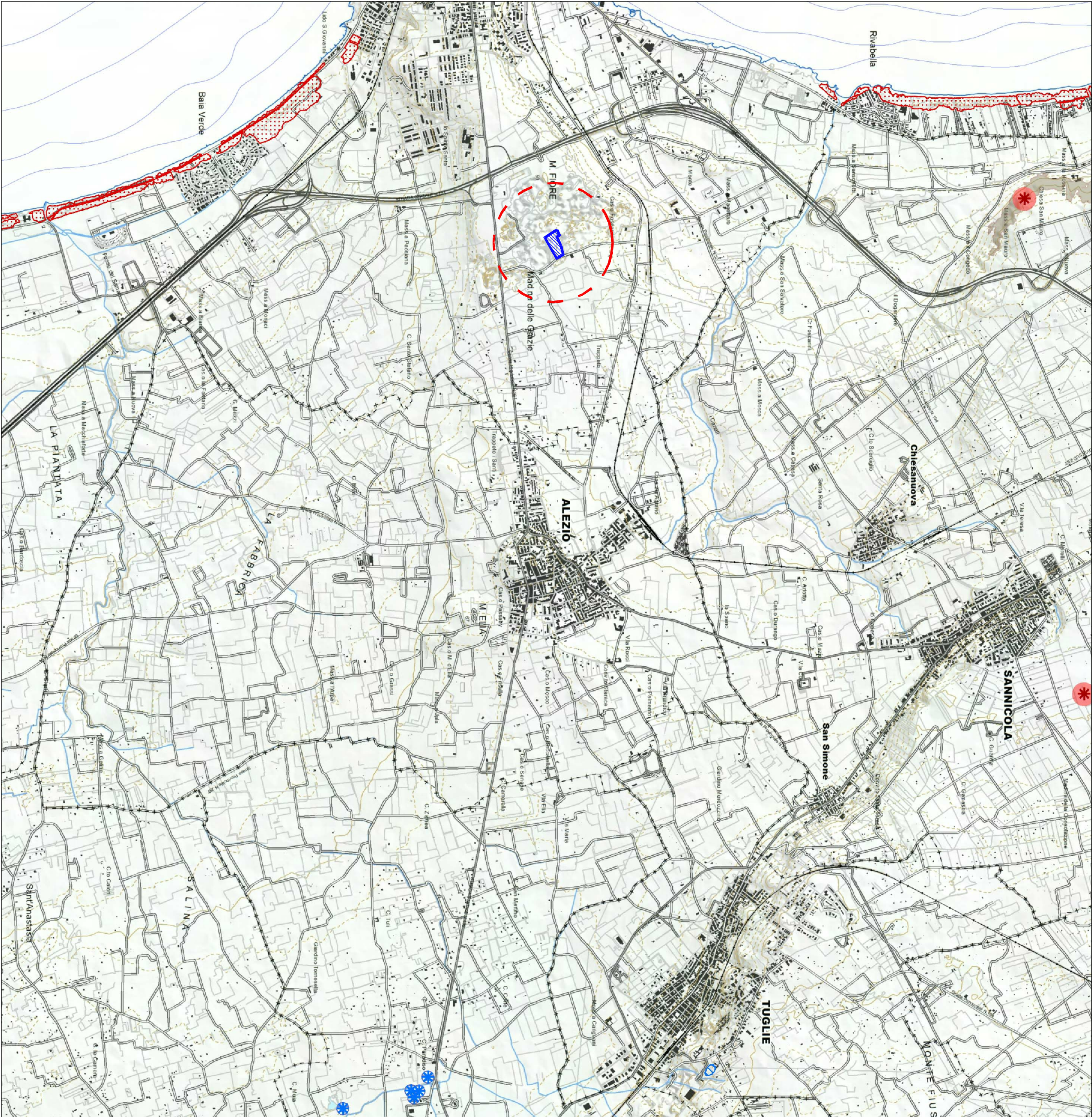
STRALCIO DELLA TAVOLA 6.1.1: COMPONENTI GEOMORFOLOGICHE - scala 1: 25.000
