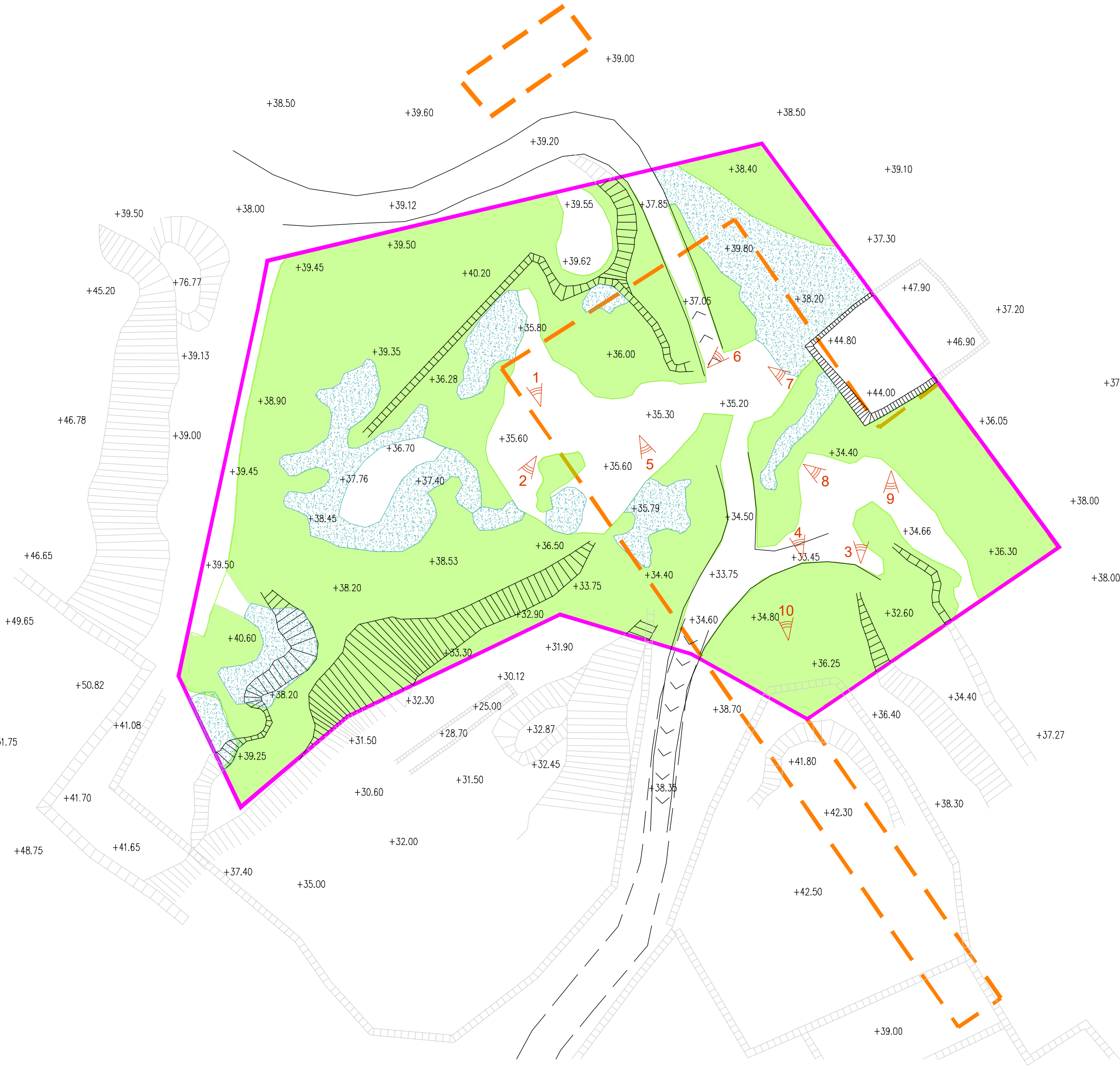
Planimetria generale con indicazione dei coni di vista - scala 1: 500
